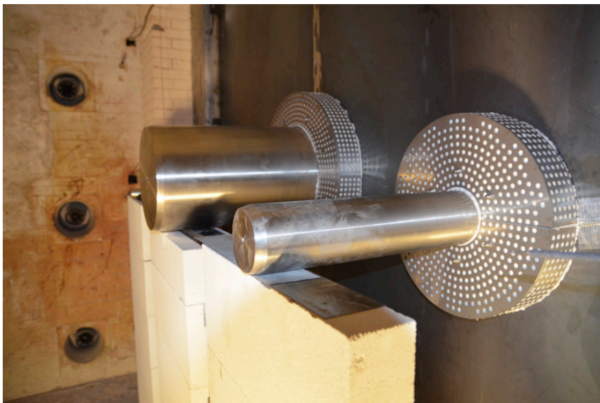
Abb. 4: Versuchsaufbau Brandtest
