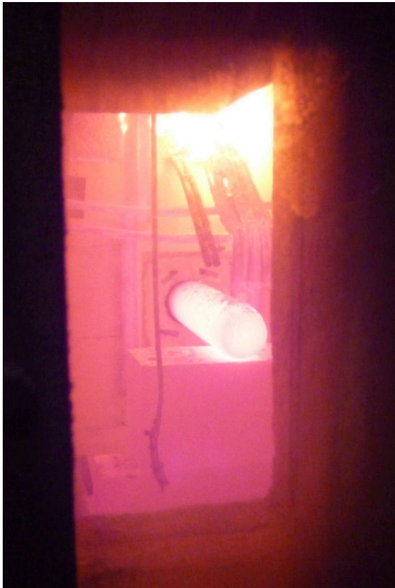
Abb. 5: Brandtest feuerfeste Schottabdichtung
